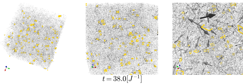
(d) Snapshot at time t = 38[J^{-1}]
