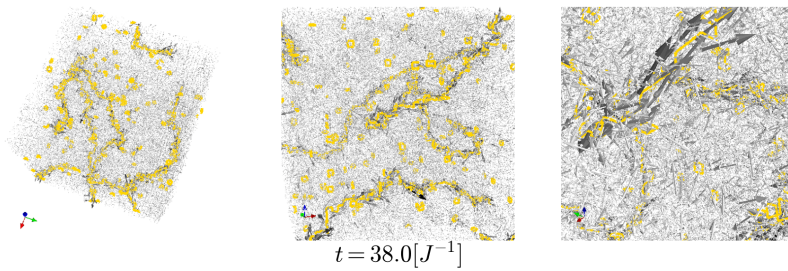
(d) Snapshot at time t = 38[J^{-1}]
